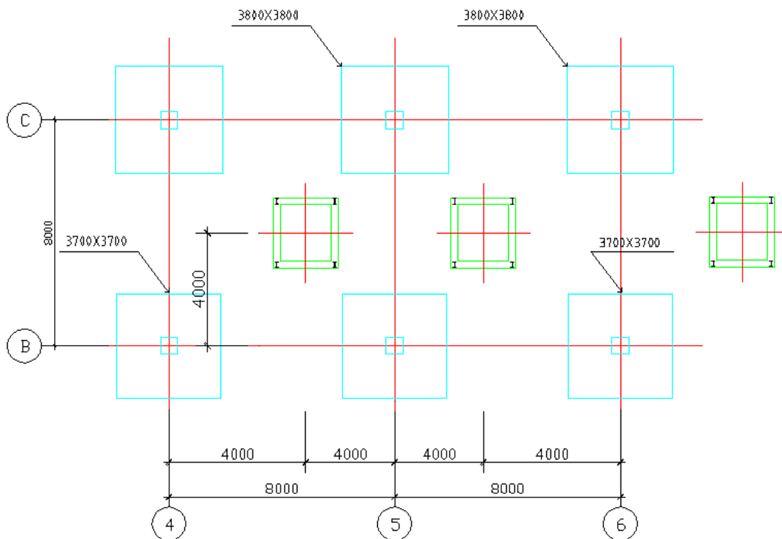
现建筑地基及新加电梯定位图
