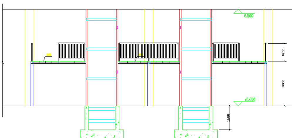
剖面示意图
